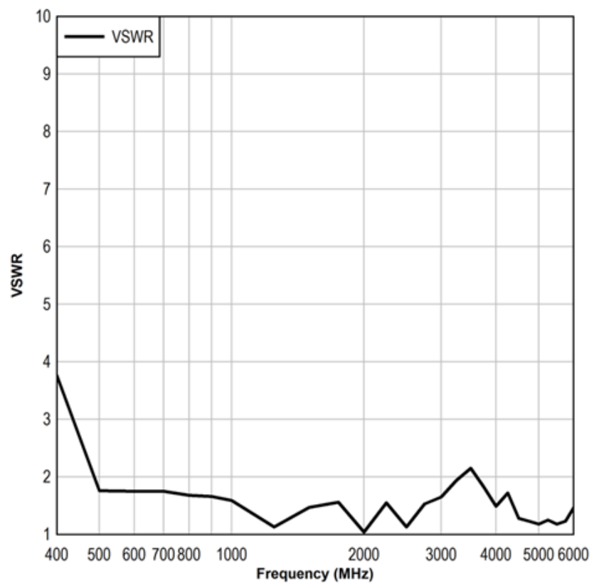
3119 VSWR
